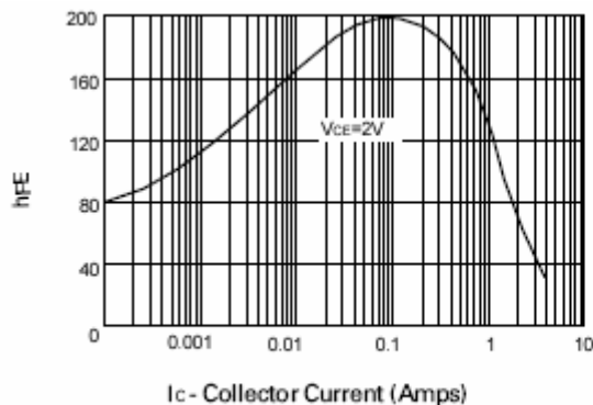
h_{FE} v I_C
